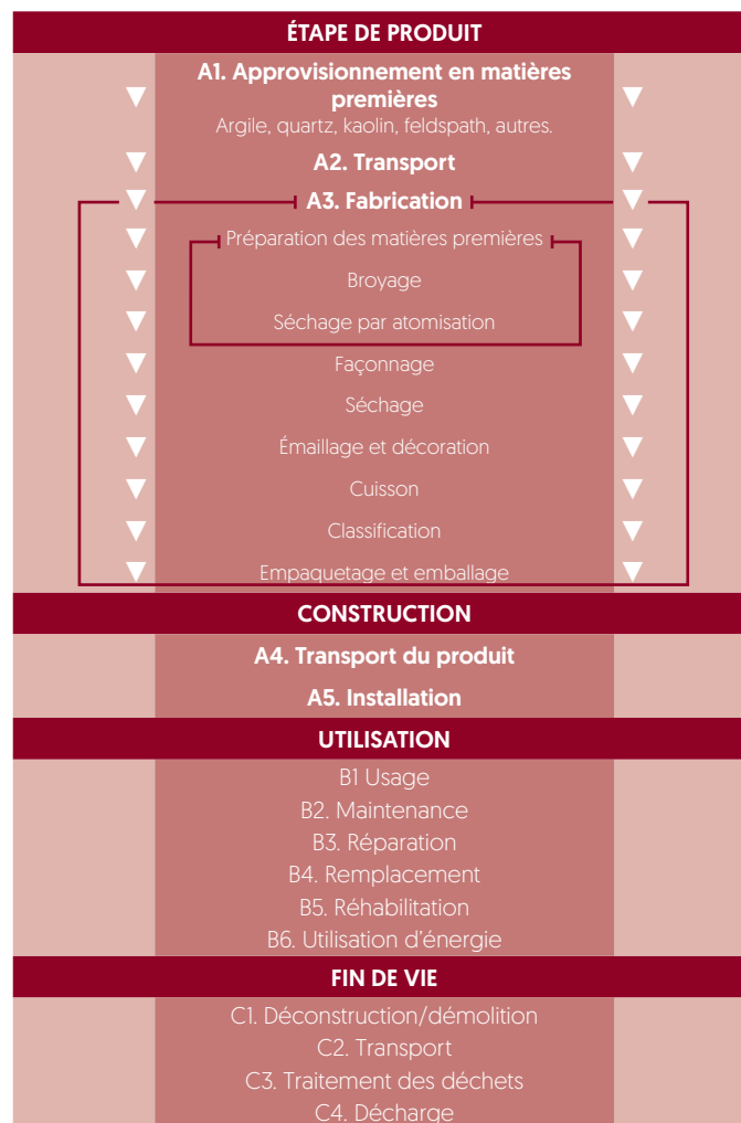
Figure 1. Diagramme avec les limites du système, les étapes et les processus pour la production d'1 m² de carreau céramique BIII 8,3 mm.
